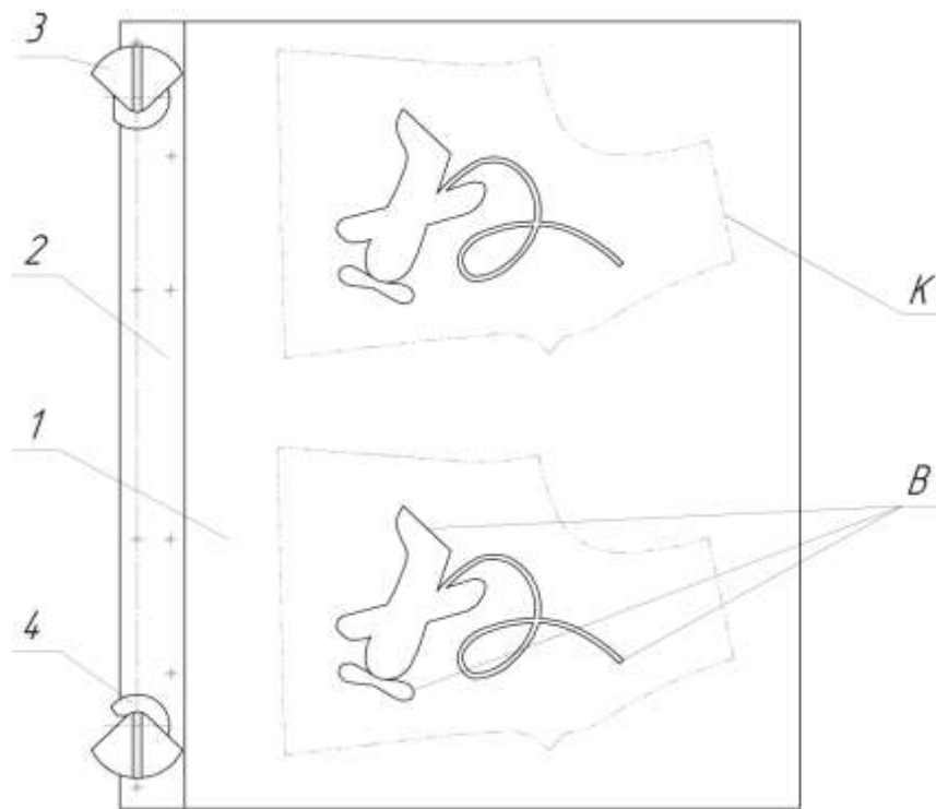
Рисунок 2 – Эскиз кассеты:
