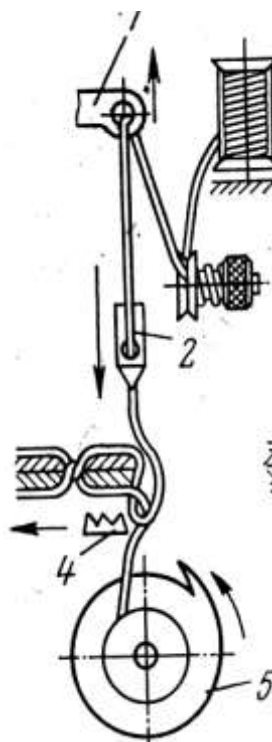
Рисунок 3 – Технологическая схема швейной машины челночного стежка
