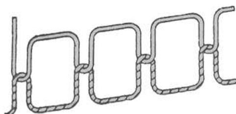
Рисунок 2 – Строчка двухниточного челночного переплетения, тип 301
