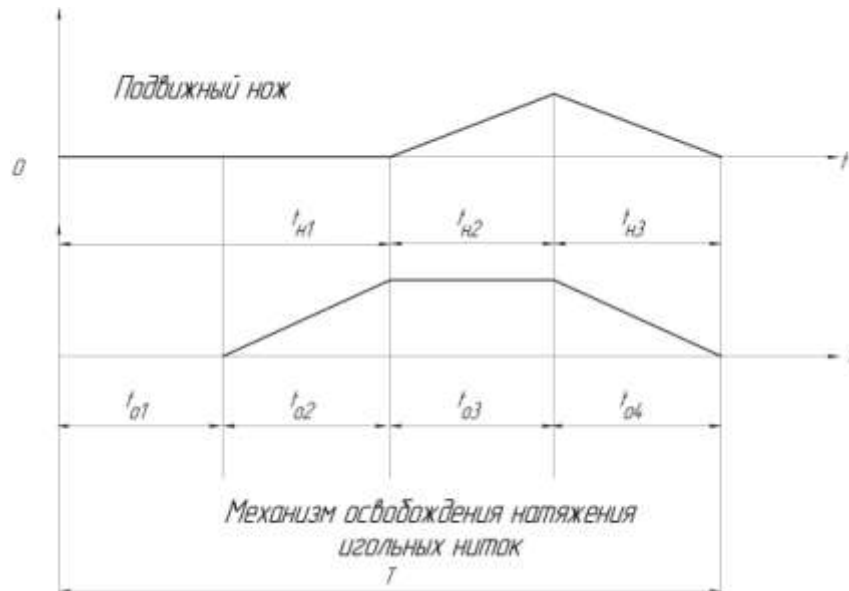
Рисунок 2 – Тактограмма
