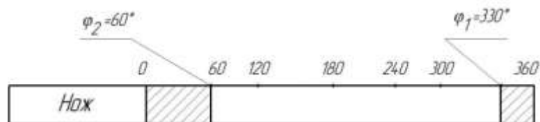
Рисунок 1 – Цикловая диаграмма подвижного ножа
