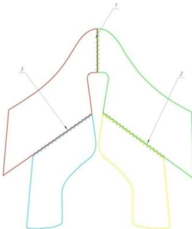
Рисунок 1 – Детали верха обуви и соединительные строчки: 1 – строчка для соединения союзки; 2,3 – строчки для соединения союзок с берцами
